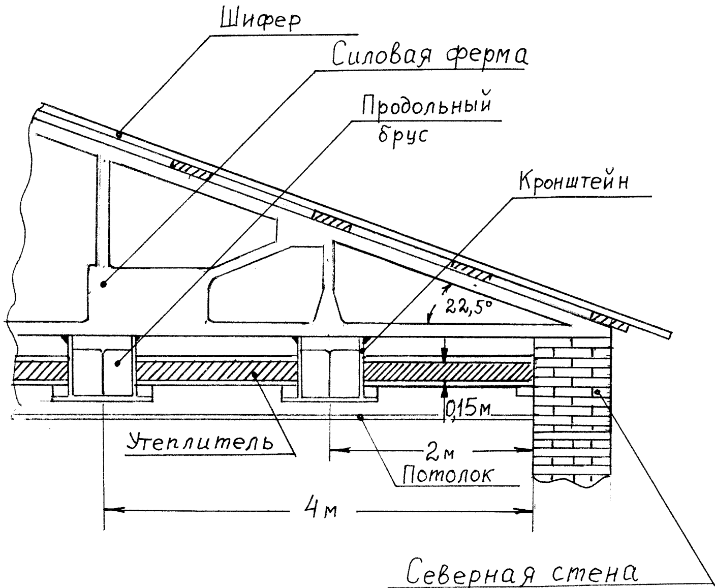
Рис. 2.34 Фрагмент устройства чердачного помещения
